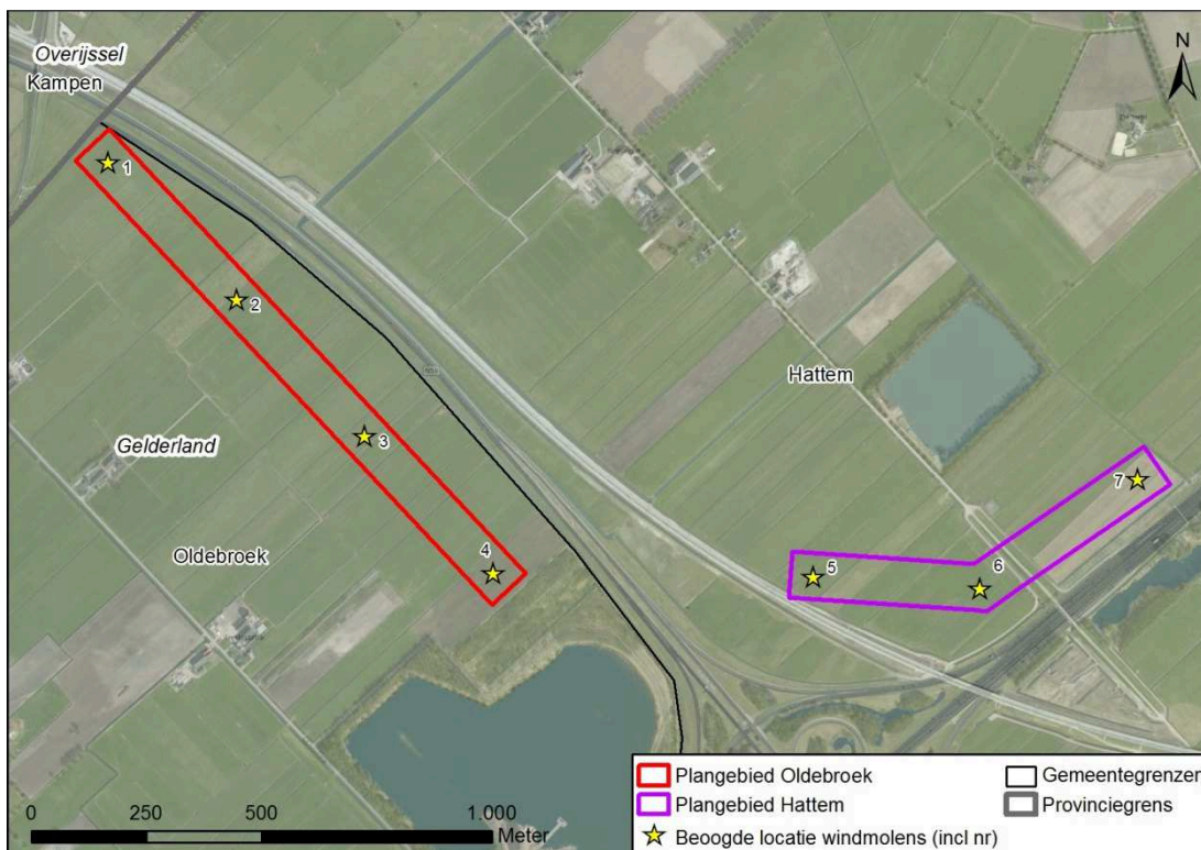
Figuur 4 Plangebied met vier windmolens Hattermerbroek en drie windmolens gemeente Hattem
