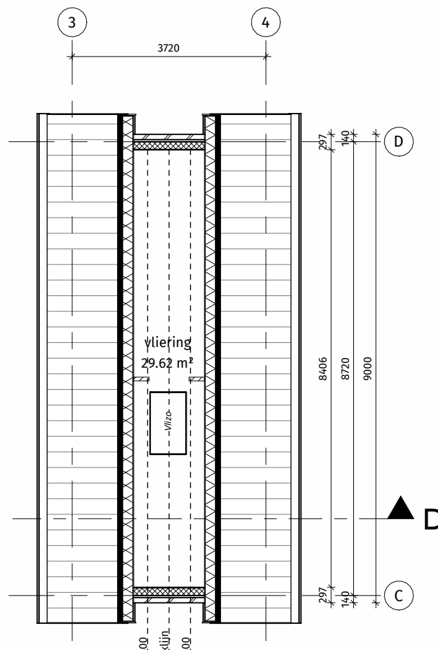
Vliering
