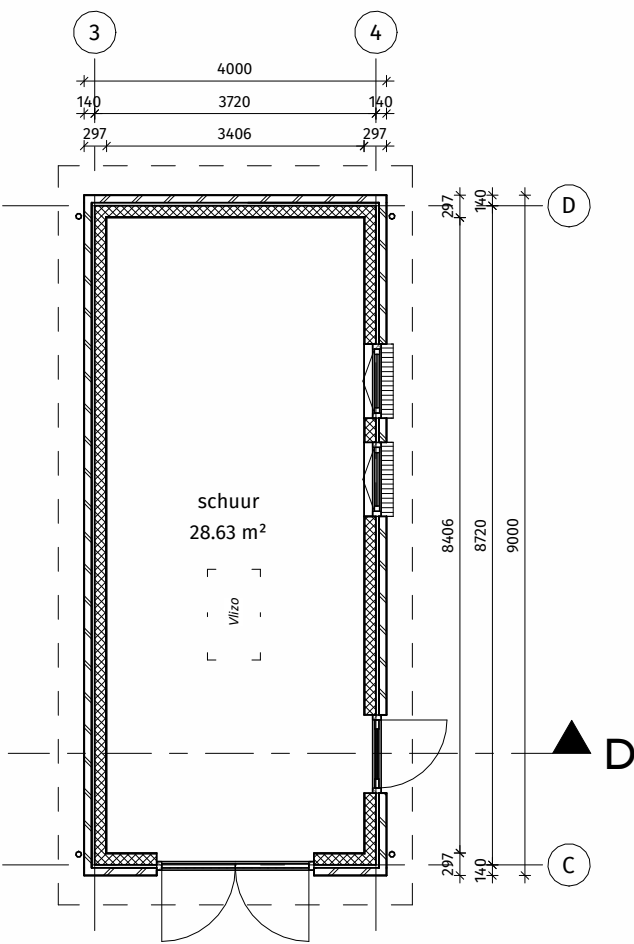
Begane grond
