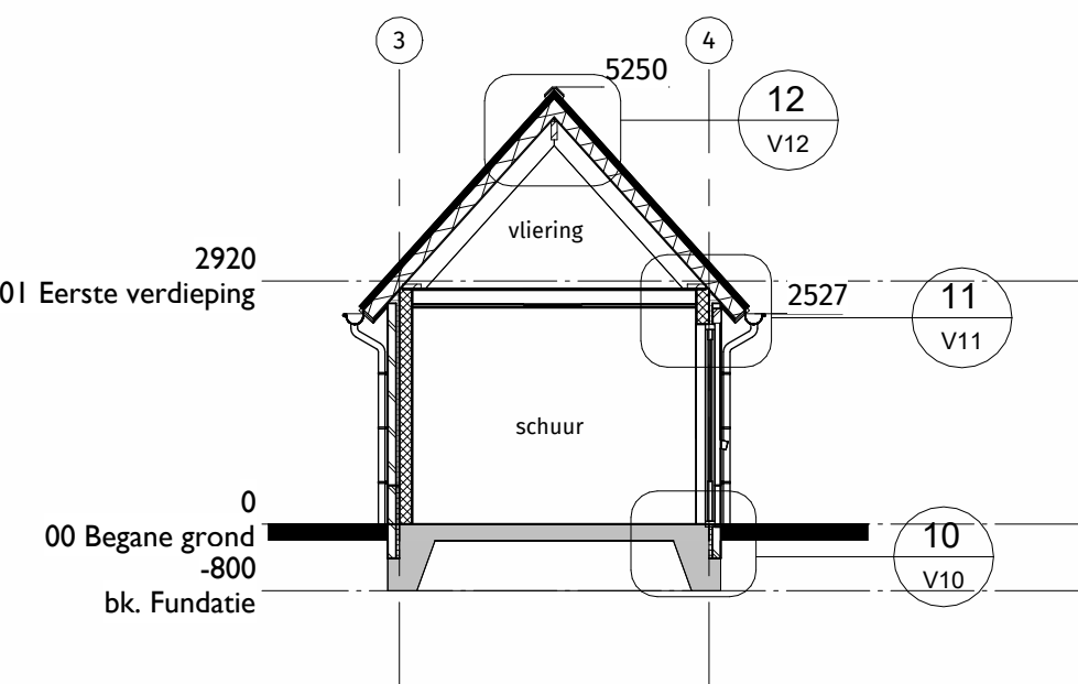
Doorsnede D
